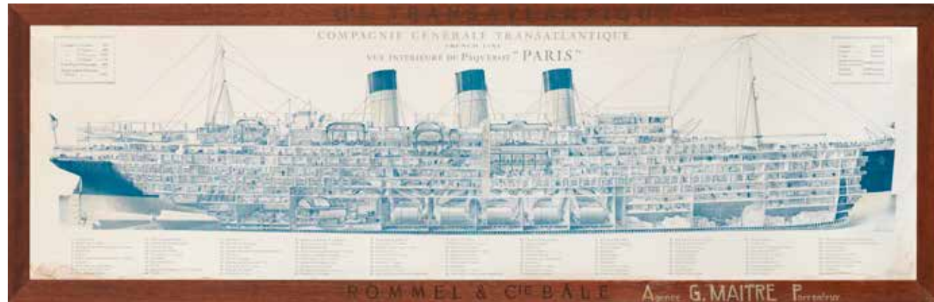
Albert Sébille, Vue en coupe du paquebot "Paris" , début des années 1920, lithographie sur papier, 32 x 108, no inv. 2022.067, don de Mme Jeanne Lovis Genève.
